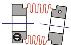
DISALLINEAMENTO ANGOLARE ANGULAR MISALIGNMENT MESALIGNEMENT ANGULAIRE
